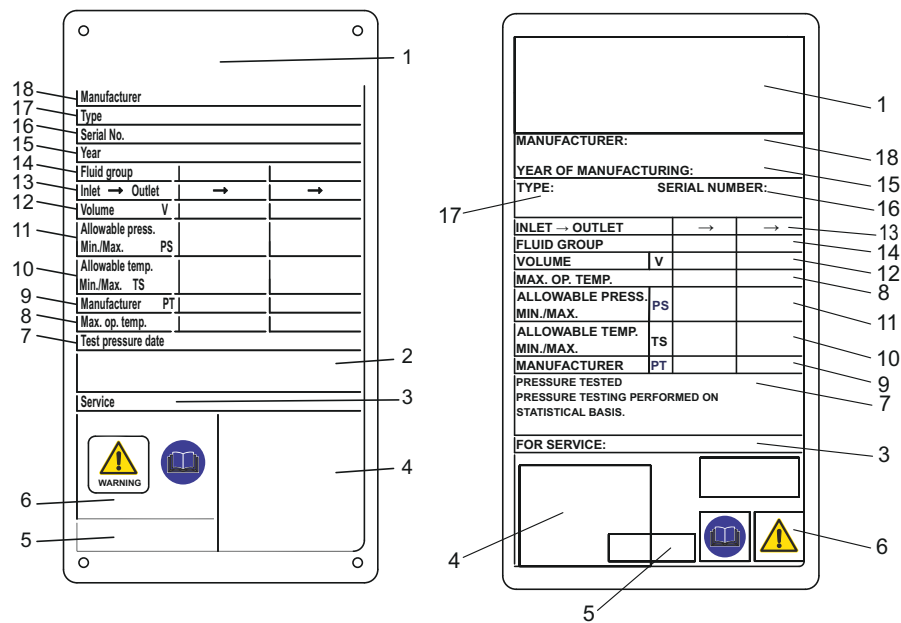
图 1：铭牌示例。
