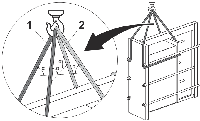
图 3：插图所示为示例设备上的吊索穿引方式。
